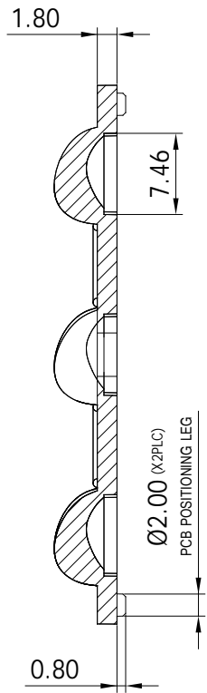
SECTION A-A
